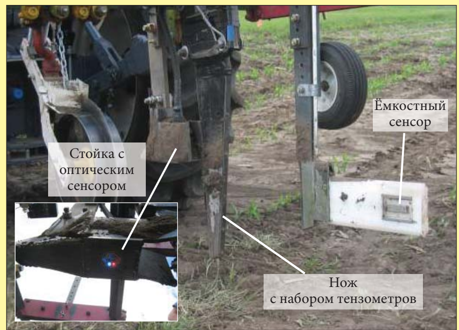
Рис. 2. Опытный образец, состоящий из механических, электрических и оптических сенсорных компонентов (Университет Небраски-Линкольна, г. Линкольн, штат Небраска, США).
