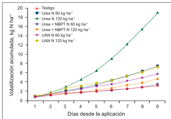
Figura 1. Emisión acumulada de N en forma de \text{NH}_3 a lo largo del periodo de evaluación en Pergamino, Argentina.
