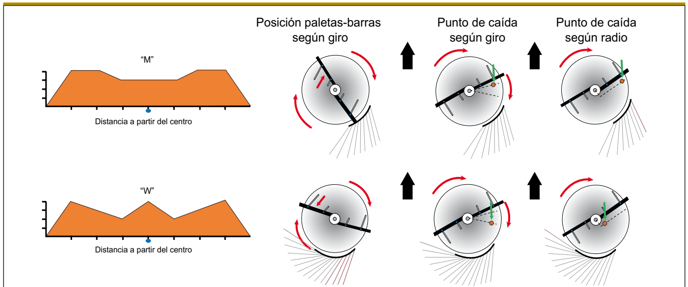
Figura 8. Modos de corrección de distribuciones de tipo M y W. Las flechas rojas indican la dirección de giro de los discos y las flechas negras, la dirección de avance de la fertilizadora. Flechas verdes y los círculos naranjas indican la posición de caída del fertilizante.
