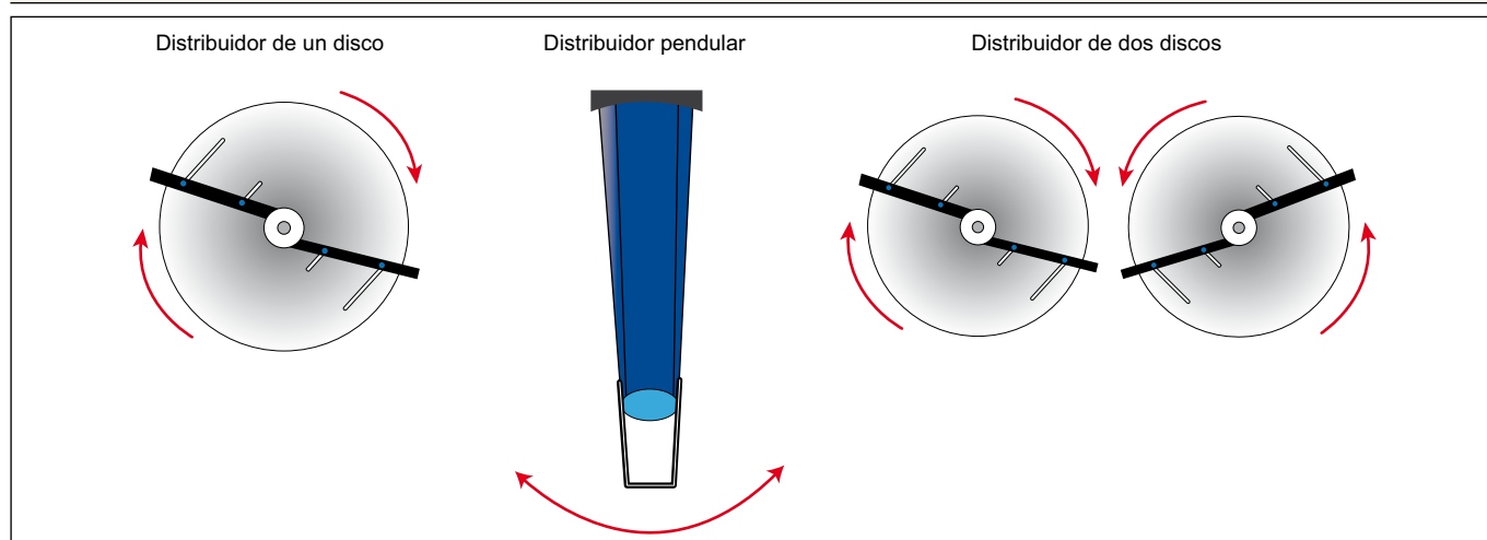
Figura 6. Distintos mecanismos distribuidores de fertilizantes presentes en fertilizadoras.
