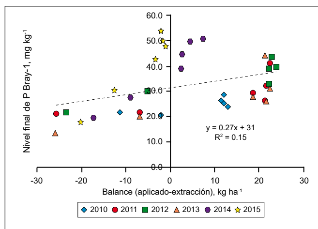
Figura 9. Relación entre el nivel final de P y el balance de P entre extracción y aplicación luego de 5 años en una secuencia continua de soja. La Trinidad, campaña 2014/15. Los valores de concentración de P y rendimiento fueron uniformados a 13% de humedad.
