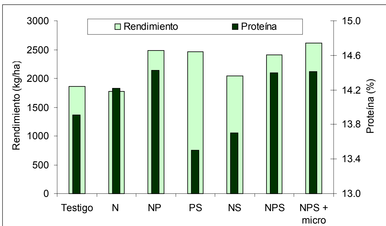
Fig. 7. Contenido de proteína y rendimiento de trigo para distintos tratamientos. Sitio Villa Eloisa 2002/03.
