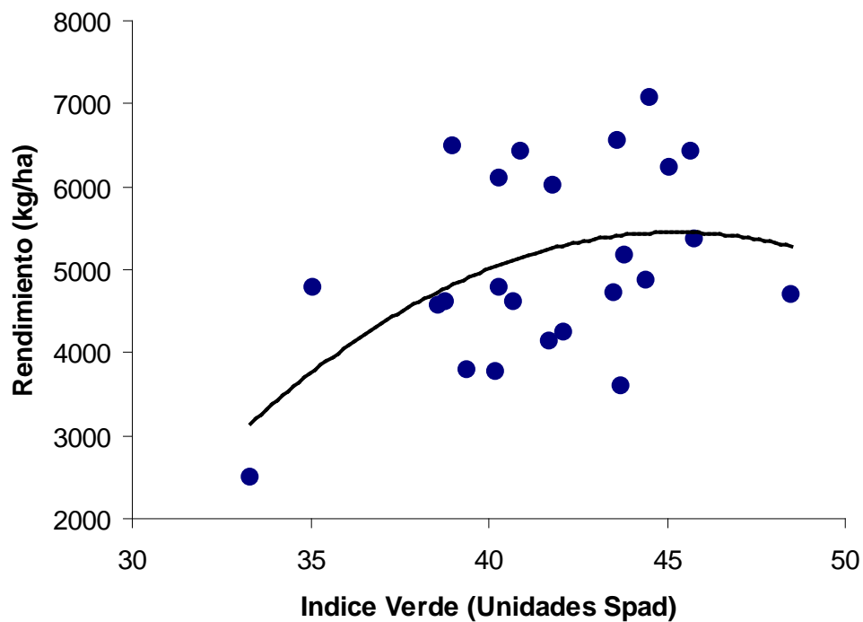
Figura 3. Relación entre Rendimiento y Unidades Spad medido en hoja bandera de trigo en el estado de Zadoks 39. La Trinidad, General Arenales. Campaña 2010/2011.
