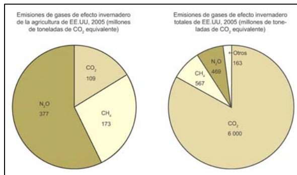
Figura 2. Emisiones de gases de efecto invernadero provenientes de la agricultura y de otras actividades en los EE.UU.
