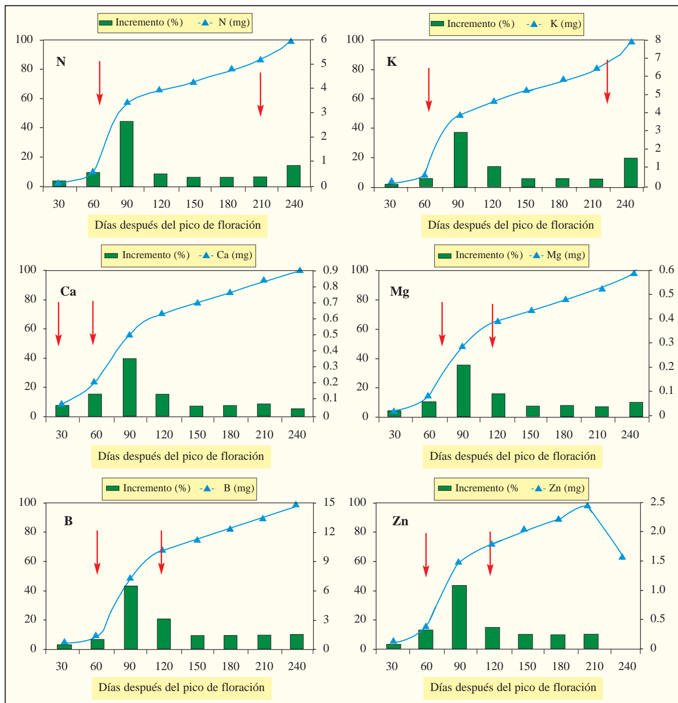
Figura 11. Curvas de absorción de nutrientes por frutos de café Caturra. Aqúares, Turrialba, Costa Rica.
