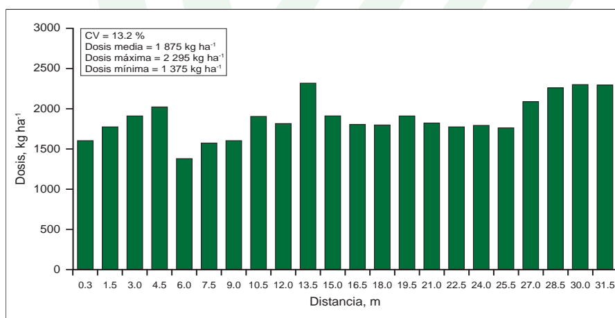
Figura 10. Perfil longitudinal de aplicación de cal con un equipo autopropulsado (Stara Hércules 24 000).
